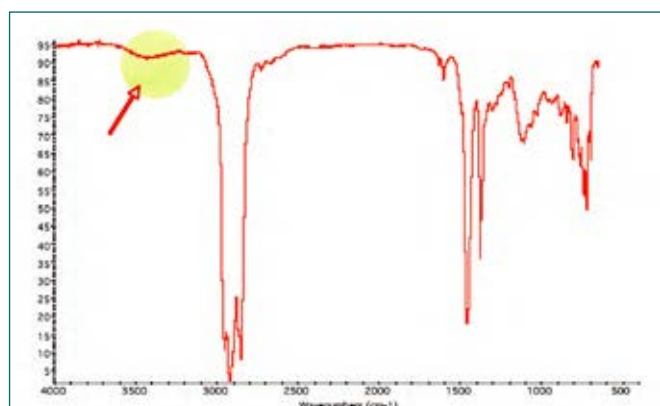
Diagramma FT-IR di un Gasolio inquinato da acqua.
