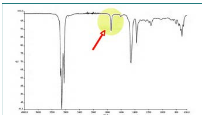
Diagramma FT-IR di un Gasolio contenente BioDiesel (8% circa).
