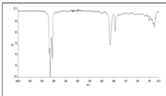
Diagramma FT-IR
