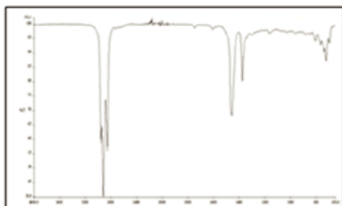
Diagramma FT-IR
