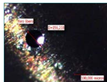
Misure fori di nebulizzazione.
